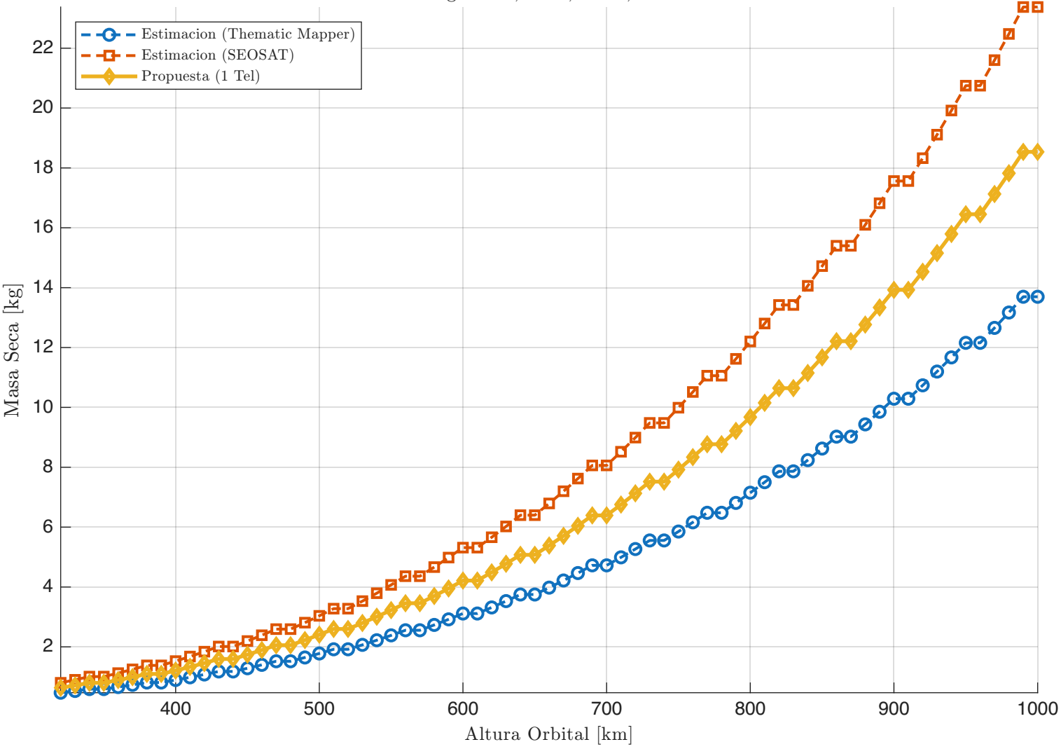
Comparativa de Masa Seca vs. Altura Config: 2 Sat, 1 Tel, Det 2, Korsch
